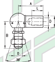
ARTICOLAZIONI A ROTULA BALL JOINTS KUGELGELENKE
