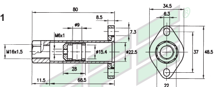
CONNETTORE KIT 001 ADAPTOR KIT 001 VENTIL ADAPTER KIT 001
