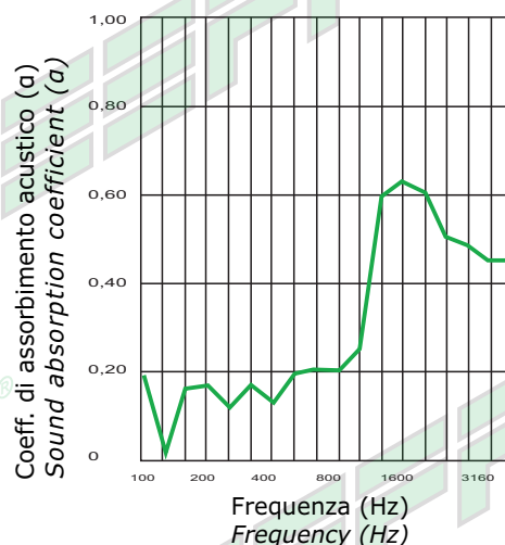
"SILENTCELL MH" (Spessore 20 mm) COEFF. DI ASSORBIMENTO ACUSTICO
